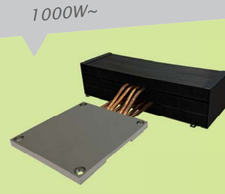
热管 / 铝鳍片
