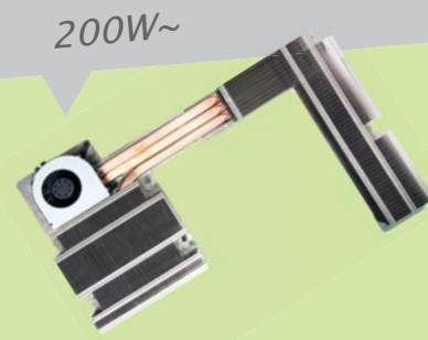
风扇 / 热管 / 铝鳍片
